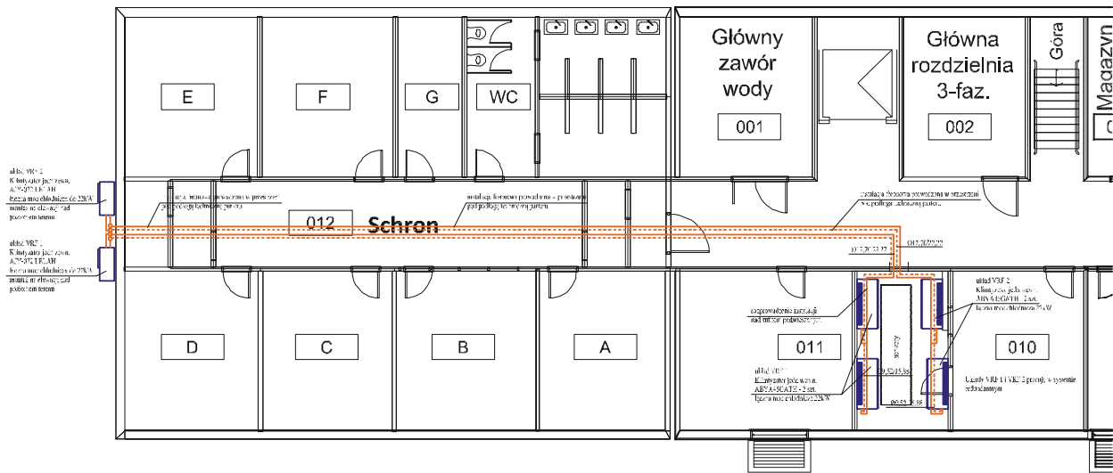
Rysunek 2 Schemat instalacji systemu klimatyzacji
