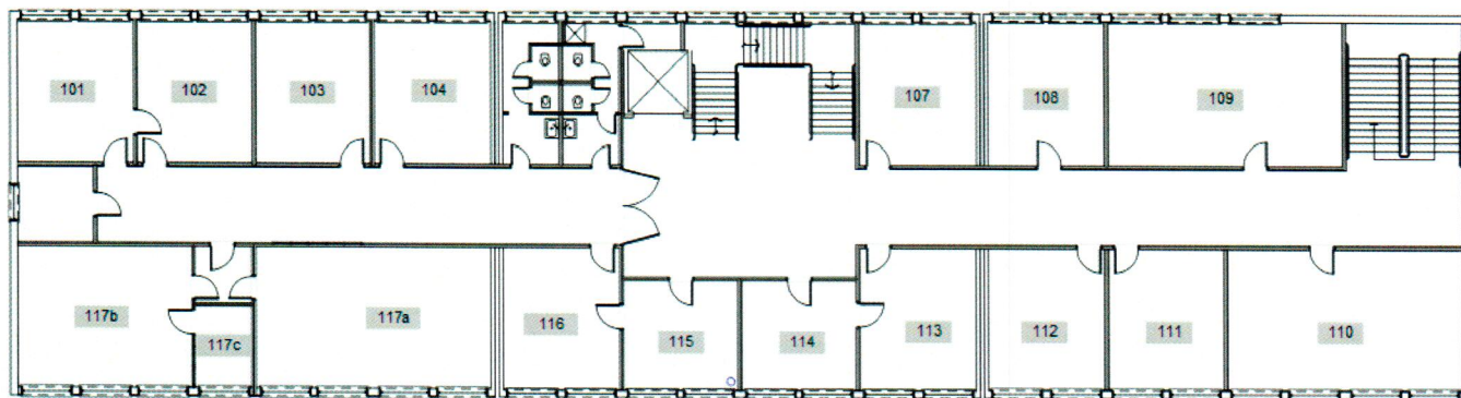
I Piętro
